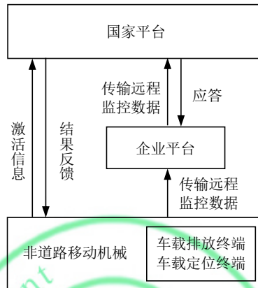
图 1 非道路移动机械排放远程监控数据流向框架
