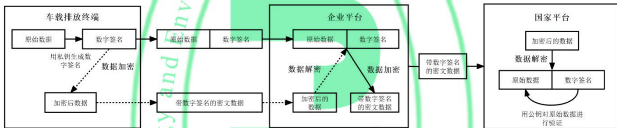
图 4 车载排放终端数据传输流程
