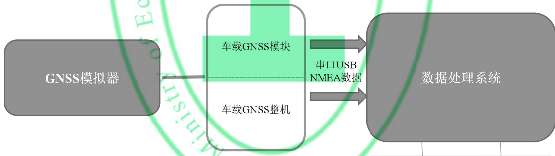
图 A.1 传导测试示意
