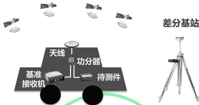
图 A.3 导航定位精度测试示意
