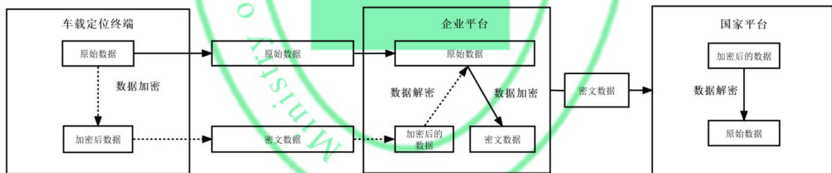
图 5 车载定位终端数据传输流程
